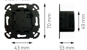
Steckmodul
